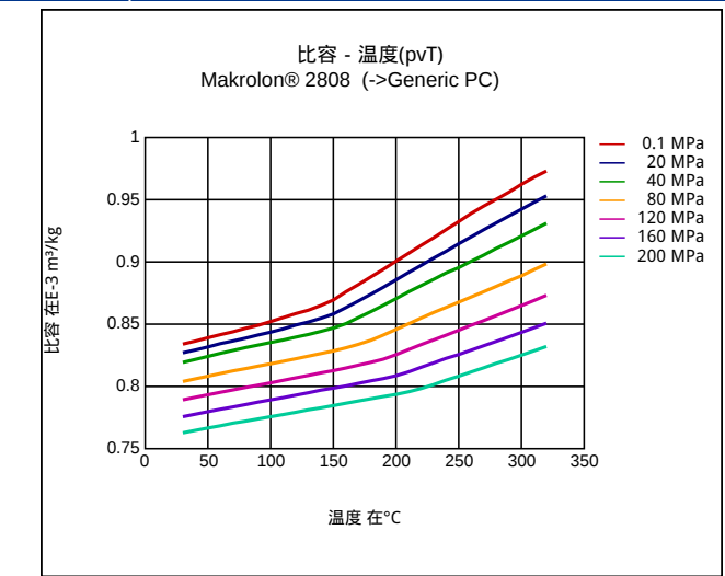
比容 - 温度(pvT)
